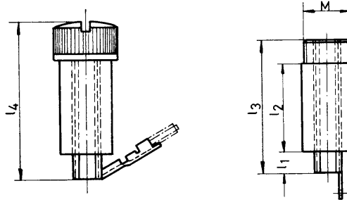
Type KK...-A
