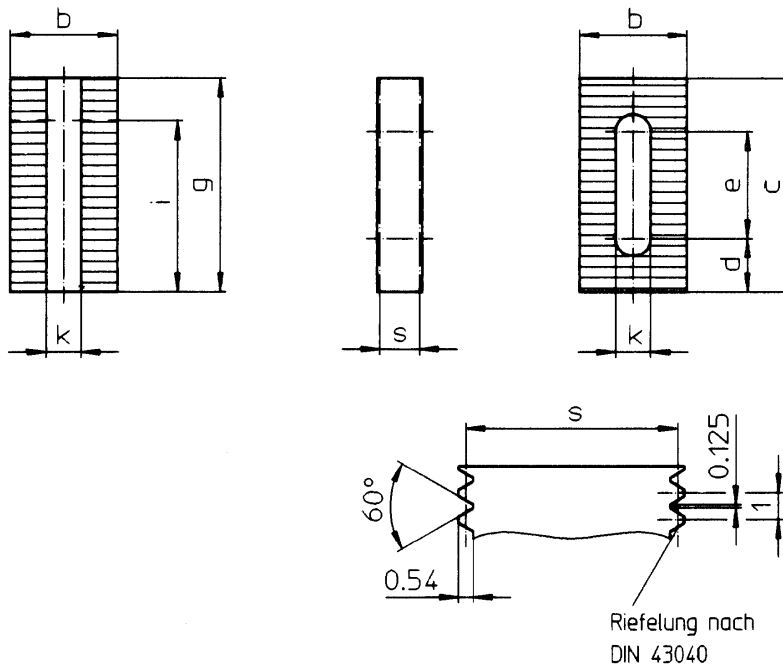
Halter/Holder/Porte-balai
