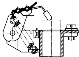
Type MES mit Kontaktblech with integrated contact finger avec lame de contact
