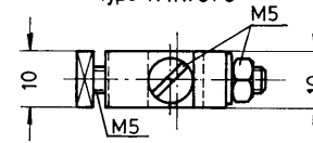
Type K1R / 10 / 10
